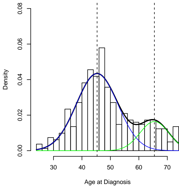
ER < 10% (n=406)
