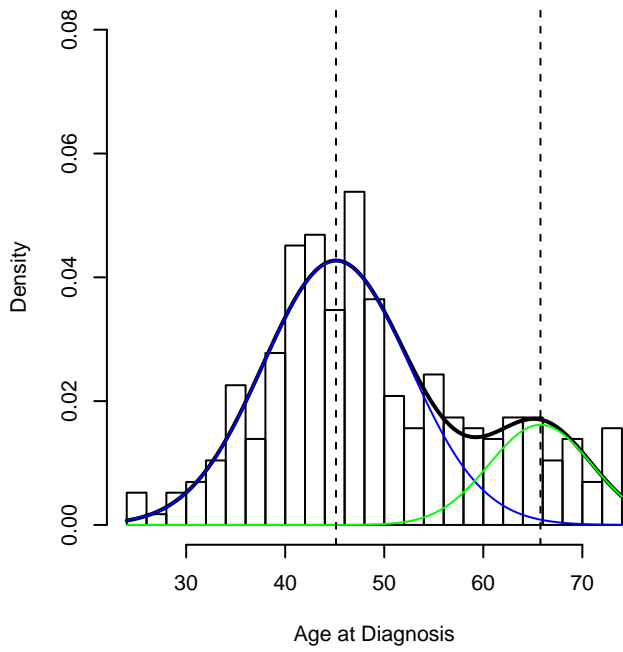
ER < 1% (n=288)
