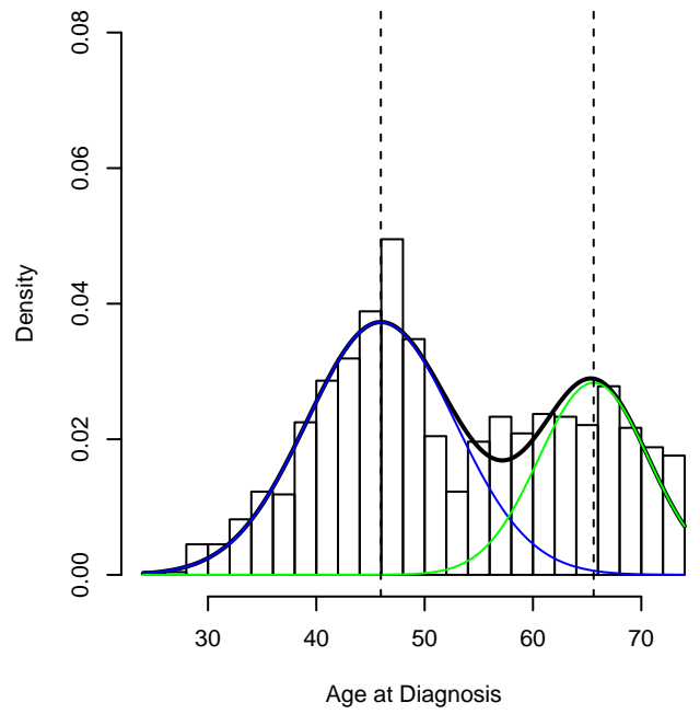
ER >= 1% (n=1222)
