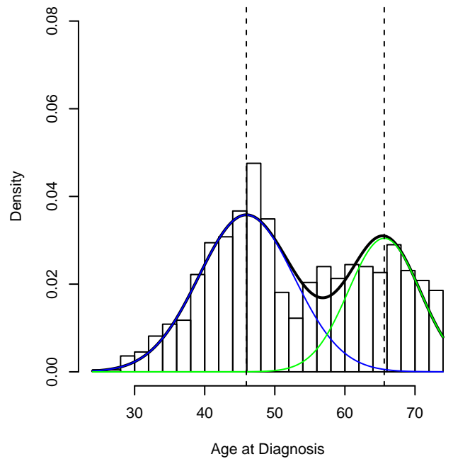
ER >= 10% (n=1104)
