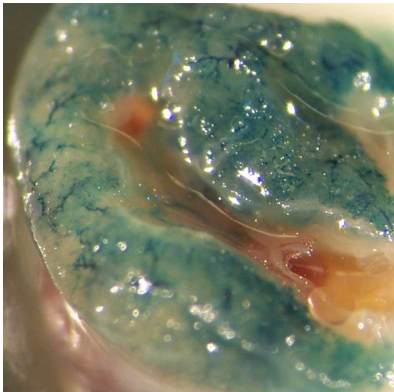
Donor VWF-lacZ
