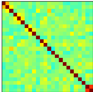
Y correlation
