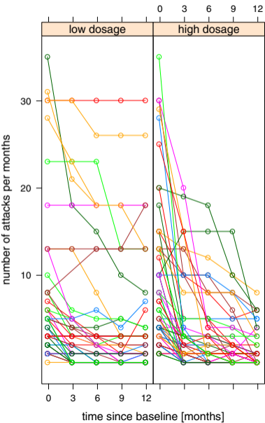
A) Original data
