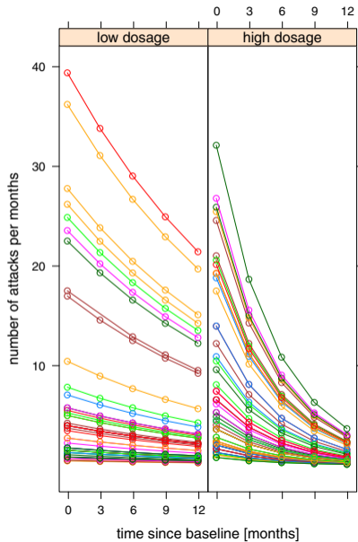
B) Poisson, I
