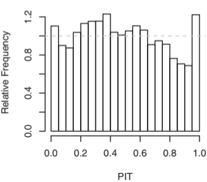
NB, I
