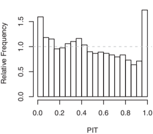
Poisson, I
