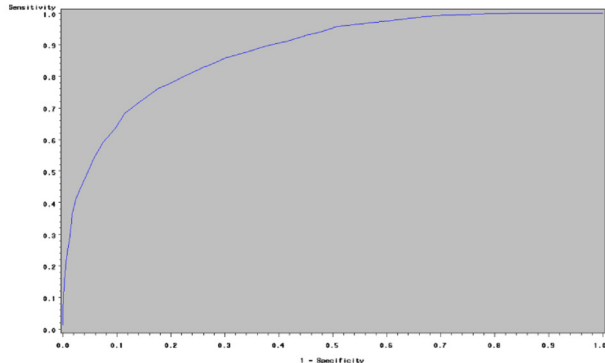
ROC Curve-Severe
