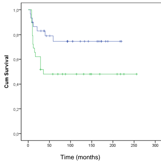
PRKCDBP
