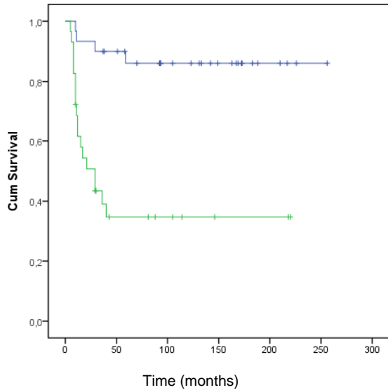
SCNN1A
