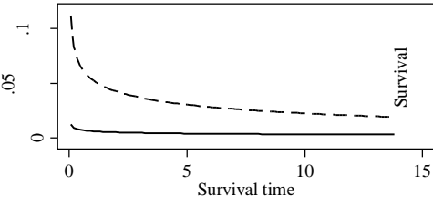
Hazard function
