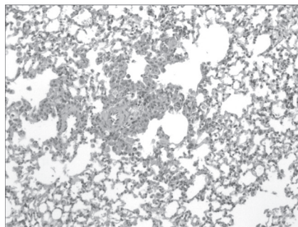
Asb + sActRIIB-Fc
