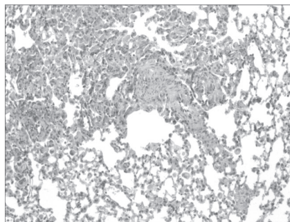
Asb
