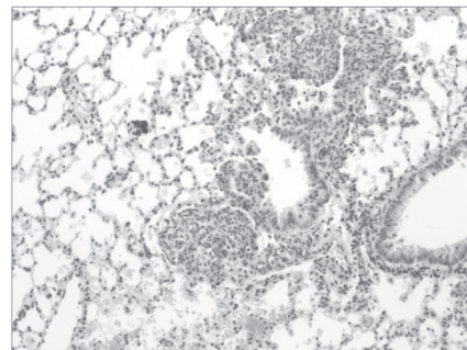
Silica + sActRIIB-Fc
