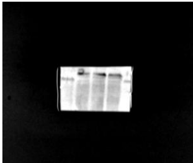
Collagen1-②
