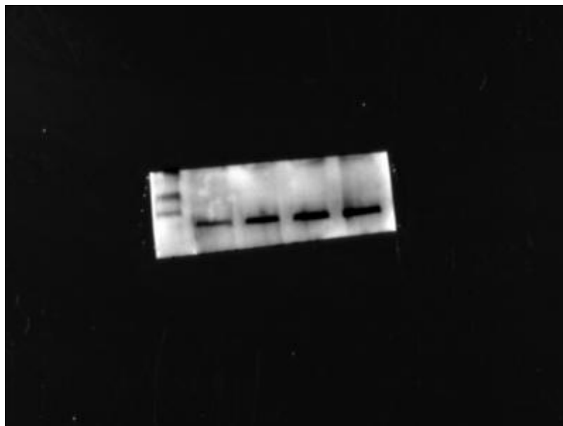
Collagen1-②
