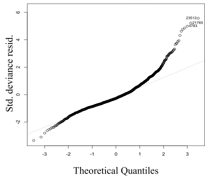
Normal Q-Q
