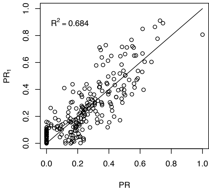
Linear Regression
