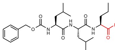
MG115
