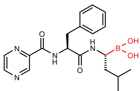
Bortezomib (Velcade)
