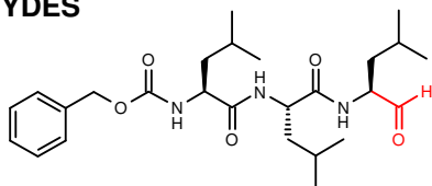
MG132
