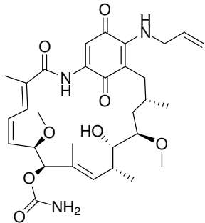
17-AAG
