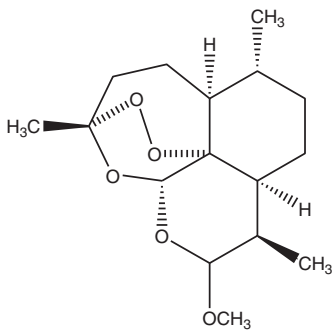
Artemether
