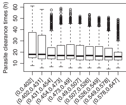
PQ k max deciles
