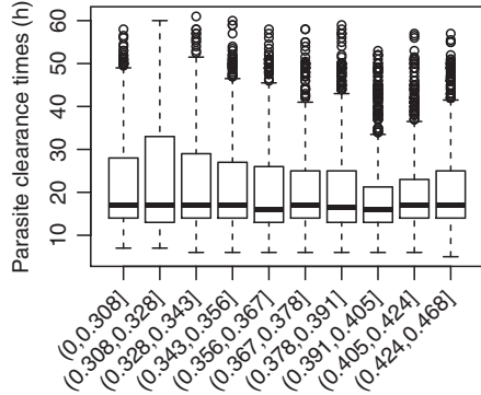
DHA k max deciles
