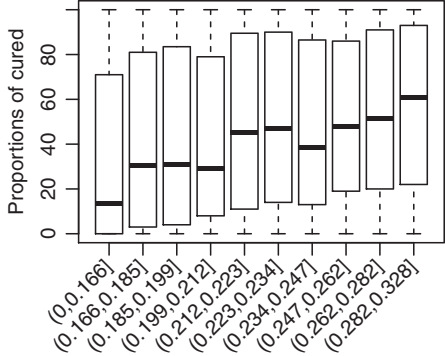
ART k_{max} deciles
