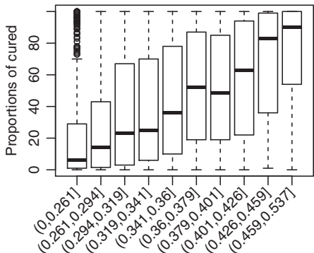
LF k_{max} deciles
