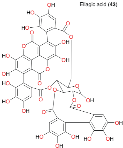
Punicalagin (42)
