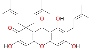
Allanxanthone C (78)
