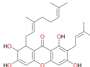
Norcowanin (82)
