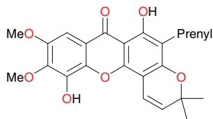
Symphonin (85)
