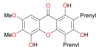
Globuliferin (86)
