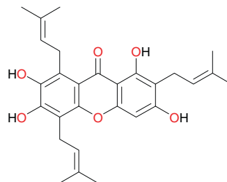
Garcinone E (90)
