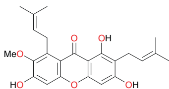
\alpha -Mangostin (89)
