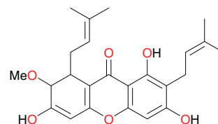
Mangostin (83)
