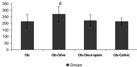
CS (nmol/mg protein)
