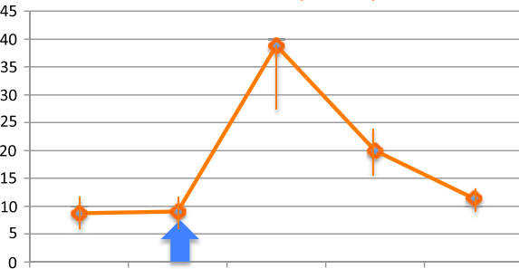
Insulin (IU/mL)
