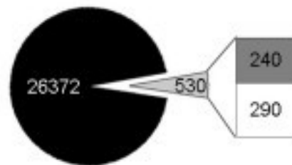
HDAC1 KD
