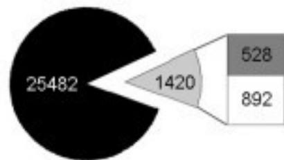
Belinostat
