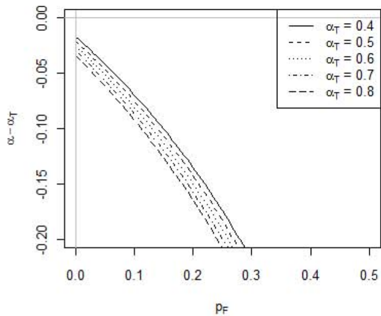
(d) p_R = 0.1, m+ - m- = 1
