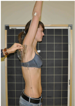
Anteflexion.
