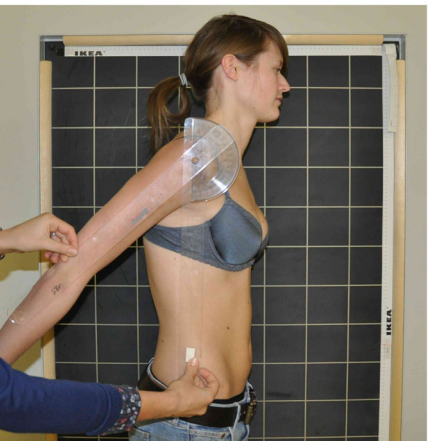
Retroflexion.
