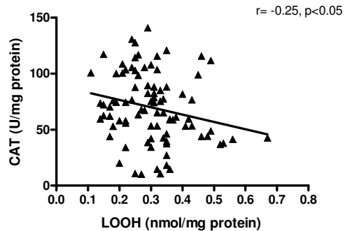
B) CAT
