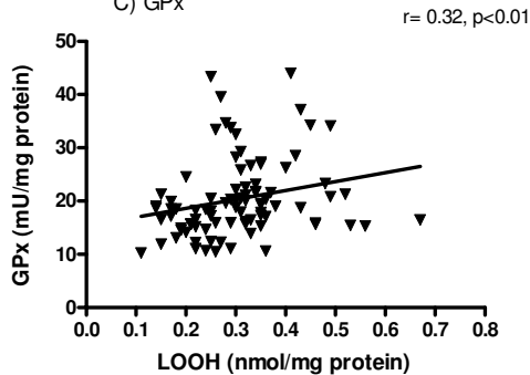
C) GPx
