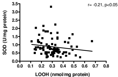
A) SOD
