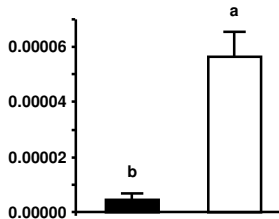
CCL2
