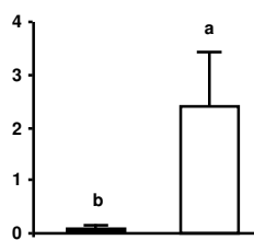
IGFBP5
