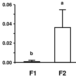
SPP1
