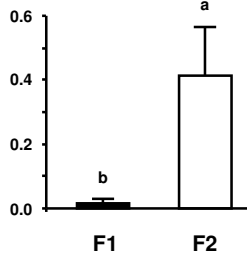
TSP2
