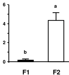
TIMP1
