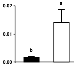
GADD45A
