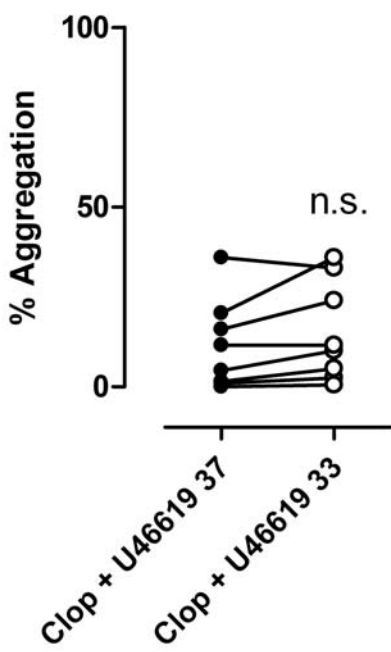
D U46619 10 \mu\text{M}
