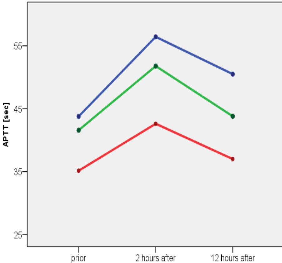
Dabigatran
