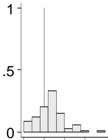
reg10==5
