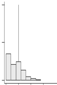
reg10==6
