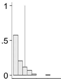
reg10==9
