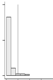
reg10==7
