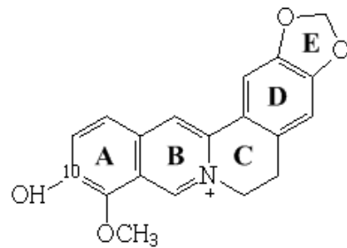
M2: thalifendine
