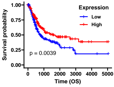
TTC28_AS1
