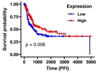
TTC28_AS1
