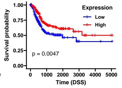
TTC28_AS1
