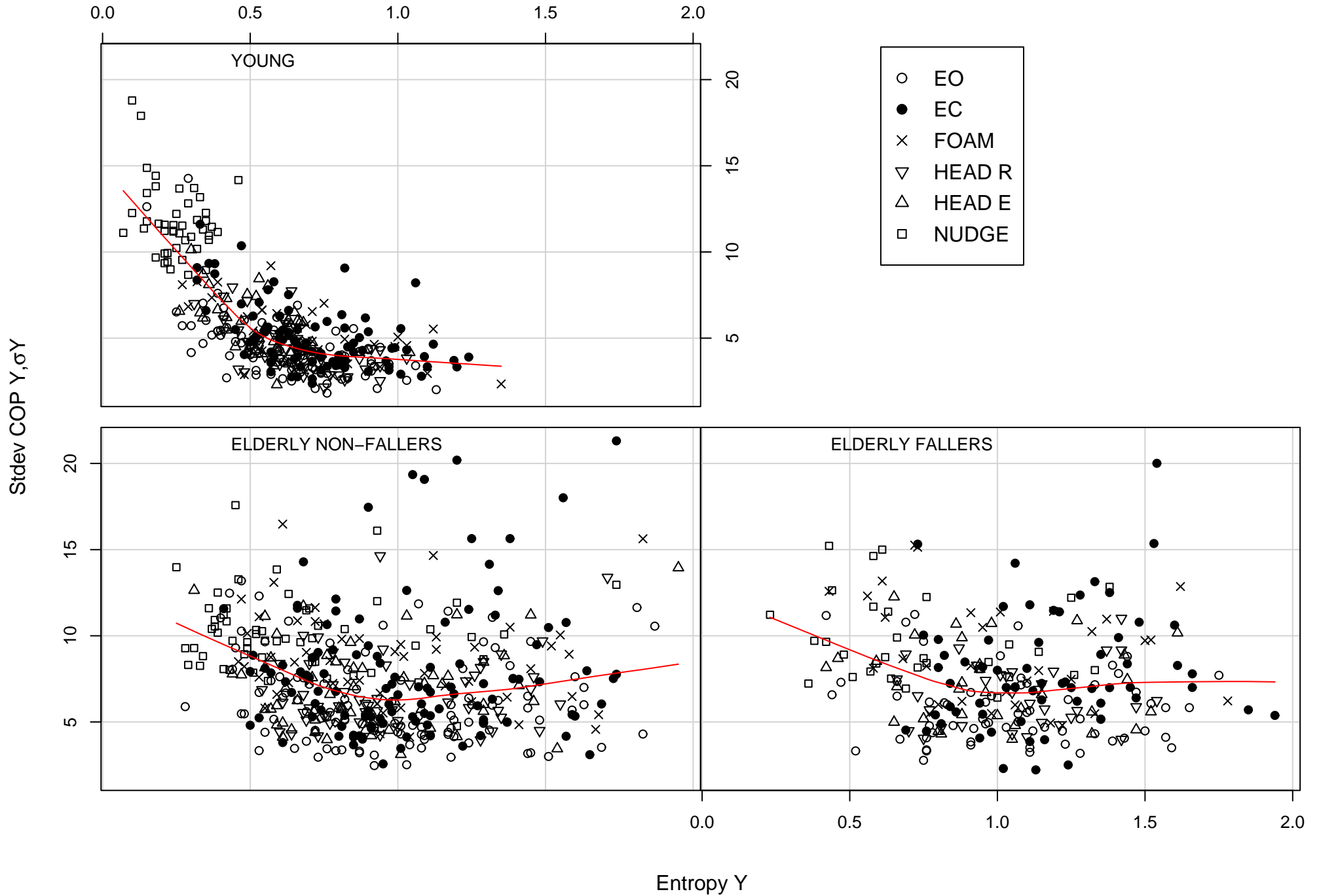
Stdev of COP Y, \sigma_Y vs Entropy Y
