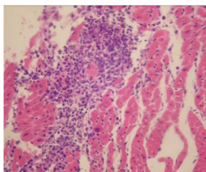
c: 7d (200×)
