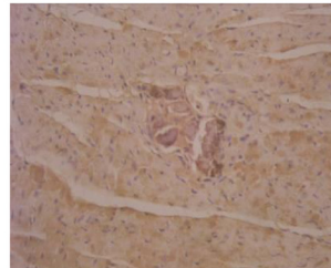
e: 40d (200×)
