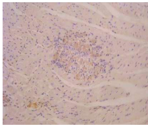
c: 7d (200×)
