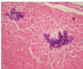
e: 40d (200×)
