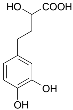
Danshensu
