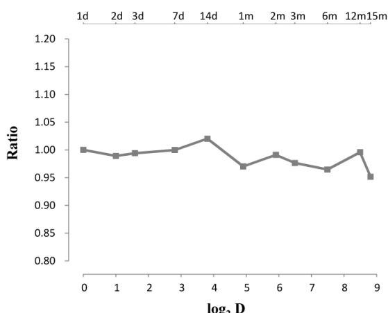
Honokiol
