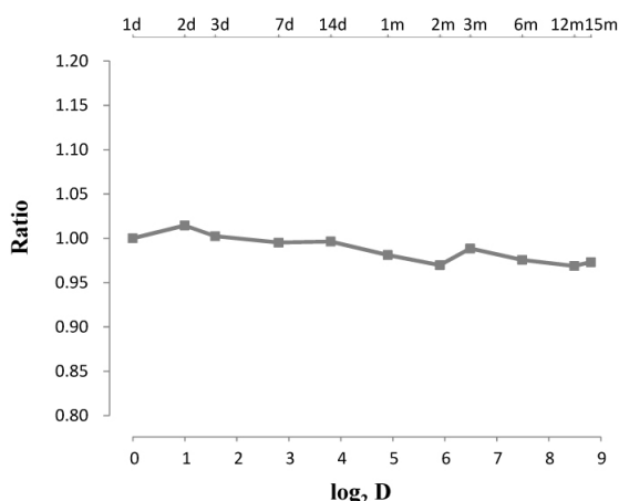
Glycyrrhizic acid
