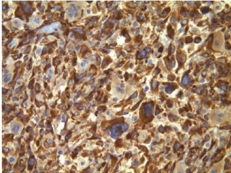
SPARC
