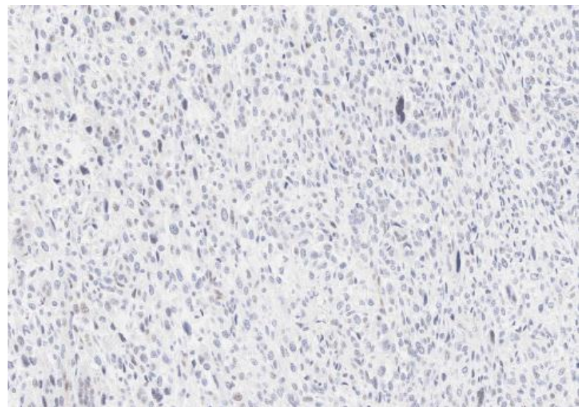
p-AKT
