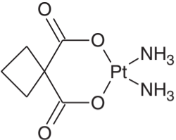
Carboplatin (CB)
