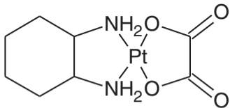
Oxaliplatin (OX)
