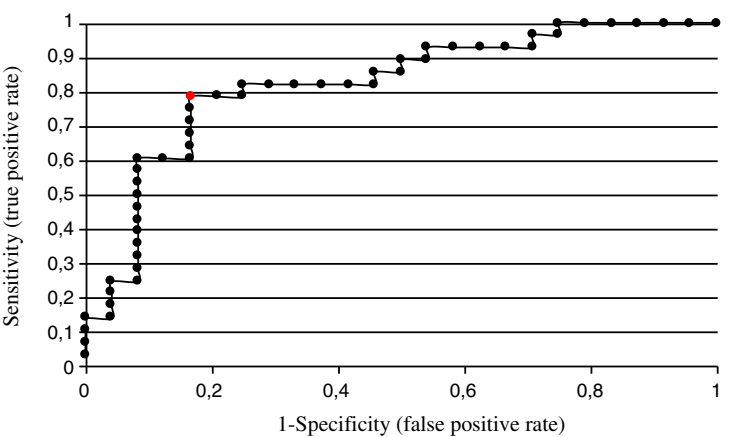
YKL-40, AUC=0.821
