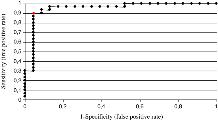
HE4, AUC=0.949
