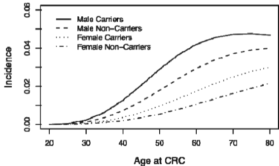
MLH1 mutation
