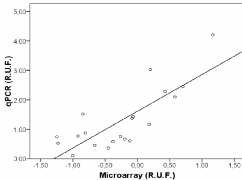
CD8 \alpha
