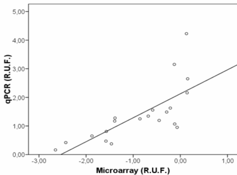
HLA-DM \alpha
