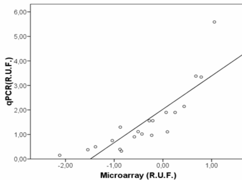
CD8 \alpha
