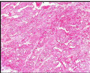
PyV mT/GTRosa
