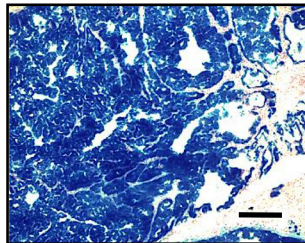
rtTA/MIC/GTRosa (+Dox)
