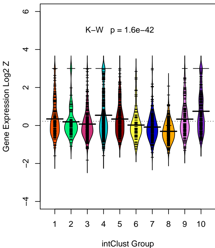
PDCD1 (ILMN_1806725)
