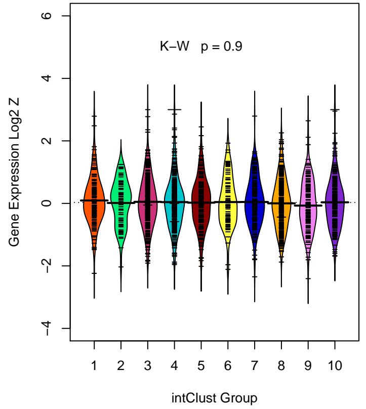
NKAIN4 ( ILMN_1813639 )
