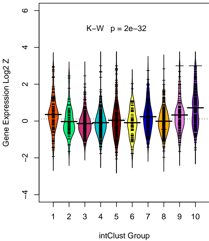
OPRS1 ( ILMN_1717925 )
