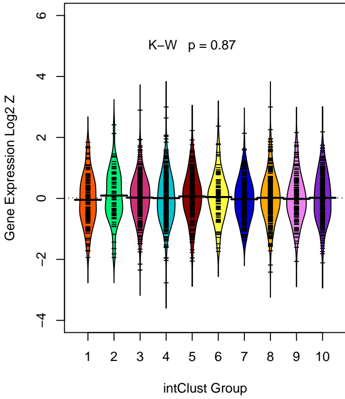
GPR182 ( ILMN_1696810 )
