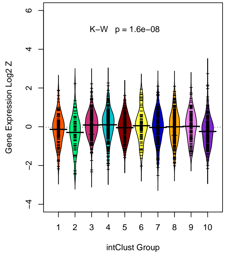
FZD2 ( ILMN_1653711 )
