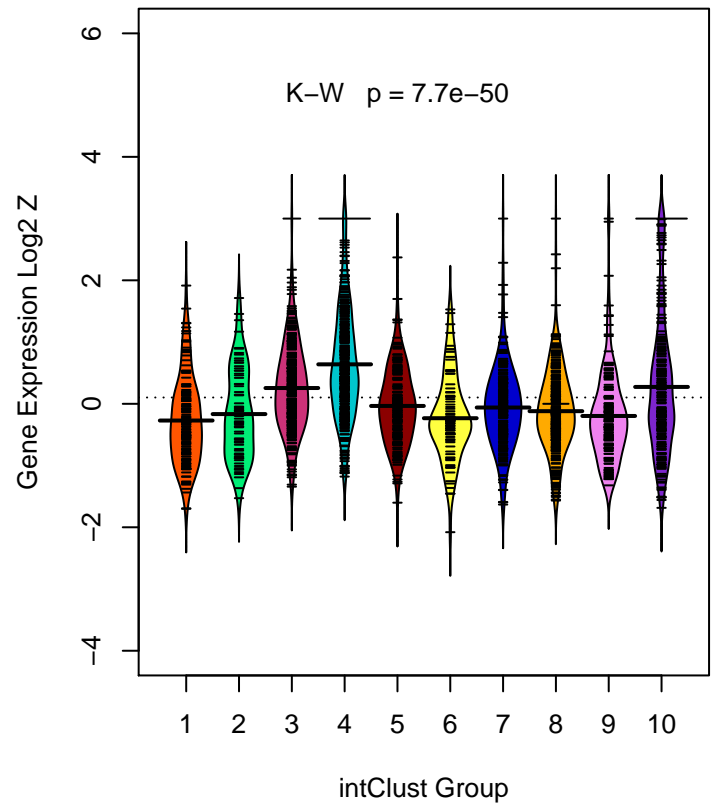
ROBO3 (ILMN_1731561)
