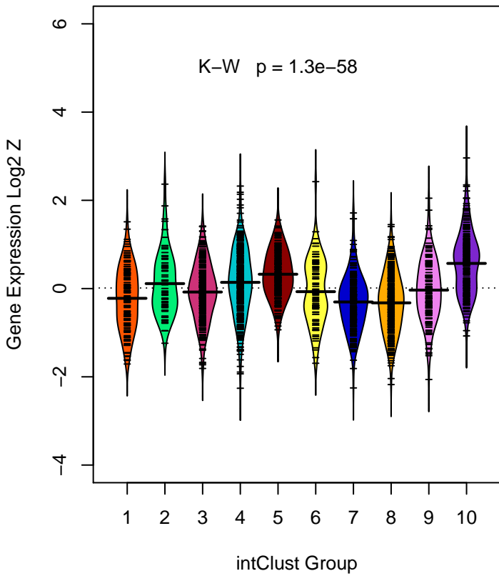
SERPINH1 ( ILMN_1751028 )
