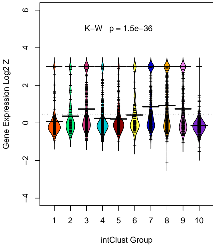
SLC6A4 ( ILMN_1683694 )
