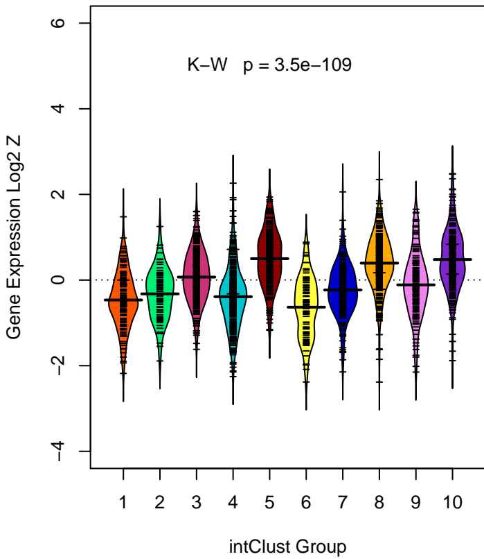
EFNA4 (ILMN_1755710)
