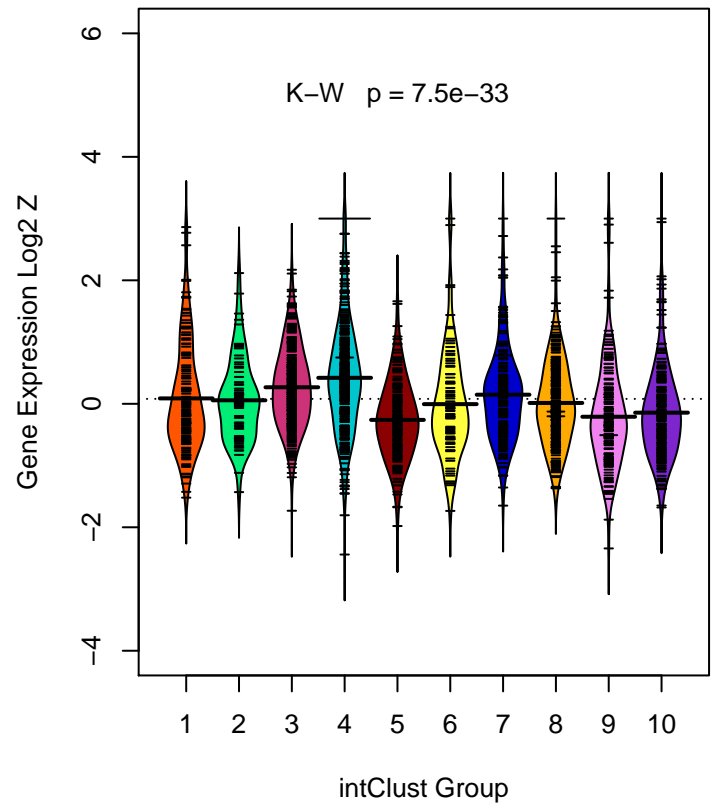
PROCR ( ILMN_1717262 )
