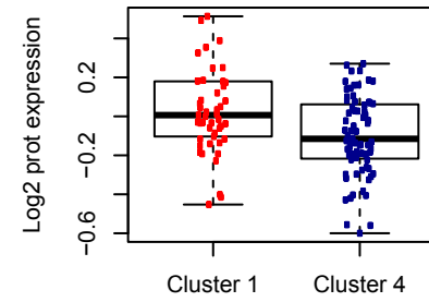
Rad51
