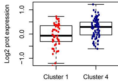
53BP1
