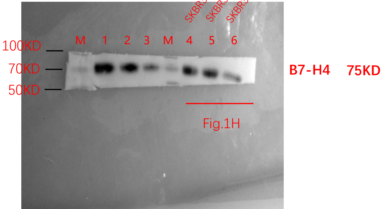
Fig.1H-(B7-H4)
