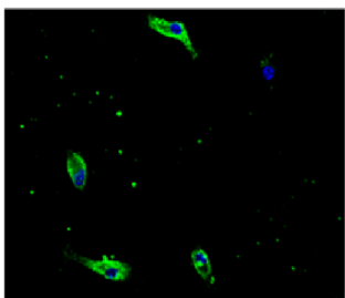
CCR2
