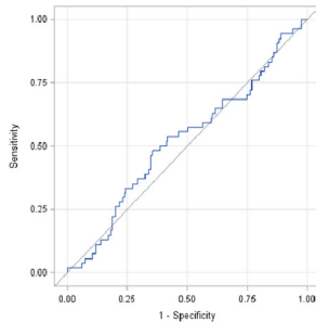
Visfatin AUC=0.52
