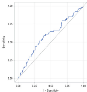
Leptin AUC=0.59
