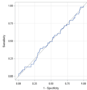
DAS28 AUC=0.50
