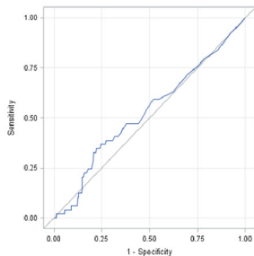
CRP AUC=0.53
