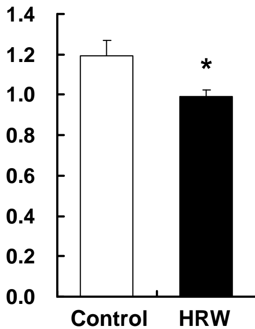
(e) Methylglyoxal
