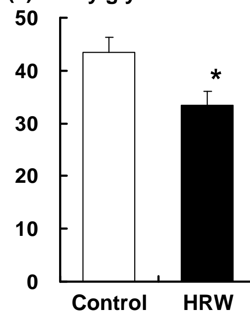
(e) Methylglyoxal
