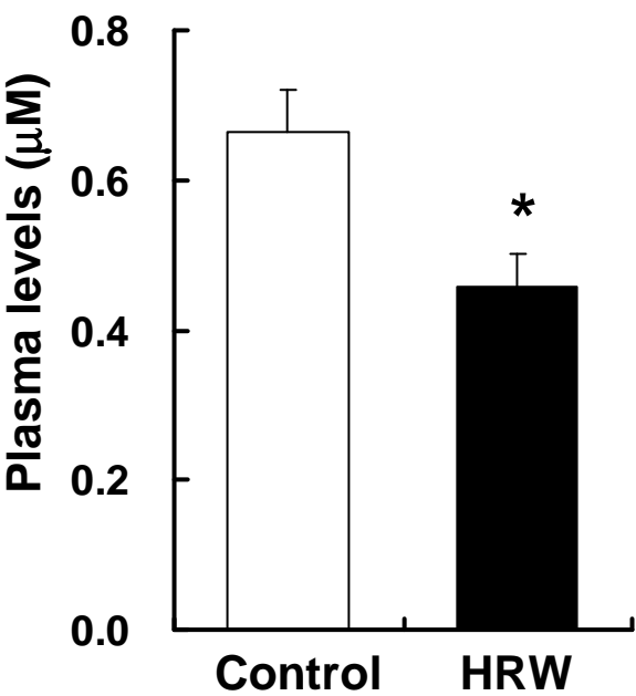
(d) Glyoxal
