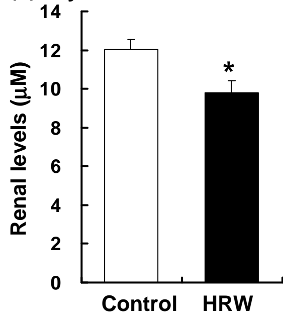
(d) Glyoxal
