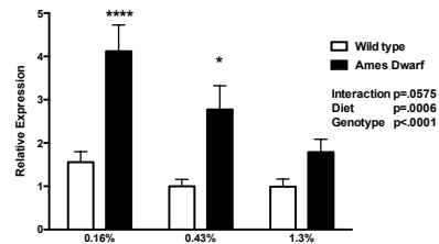
Muscle Gmmt
